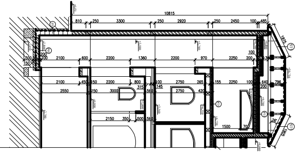
ČASTIČNÝ REZ VÝTAHOVOU ŠACHTOU
