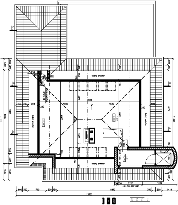
PODORNS PODKROVIA - NAVRHOVANÝ STAV
